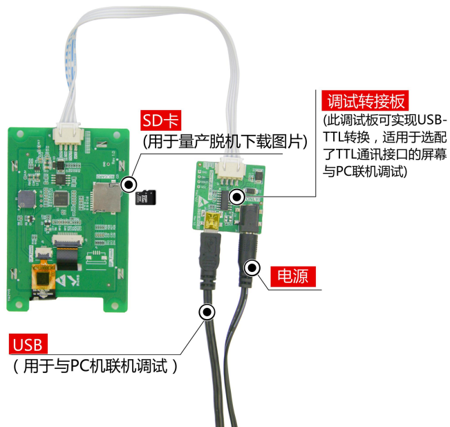
图 1-5 调试工具图
