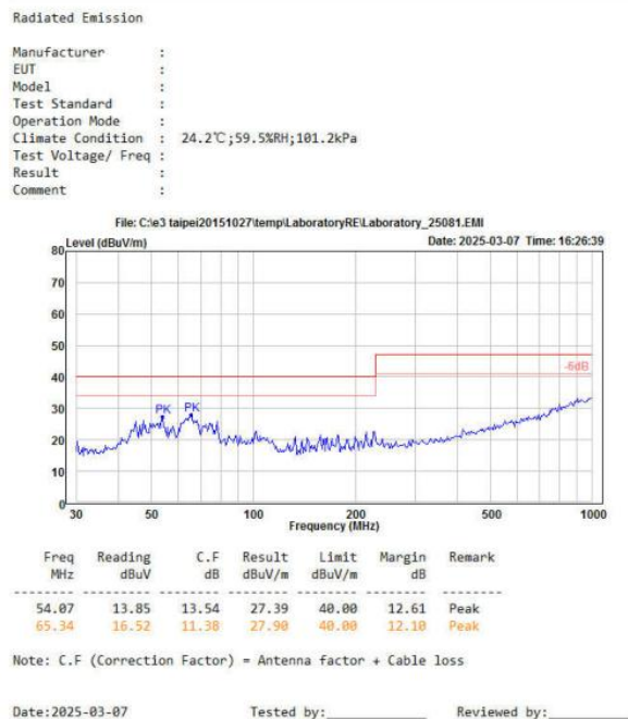
图 4-6 RE 测试垂直方向
