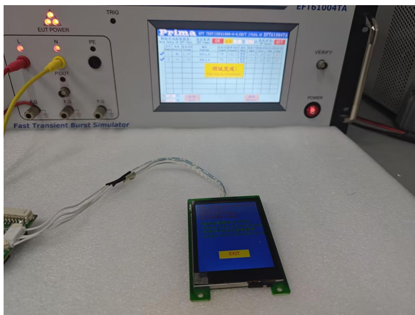
图 4-3 EFT 测试图
